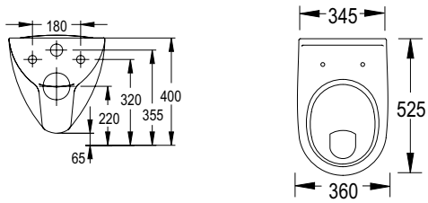
FORMAT Wand-WC Flachspüler DIN 1385-6 Ü Artikel-Nummer FO 071 619 ..
